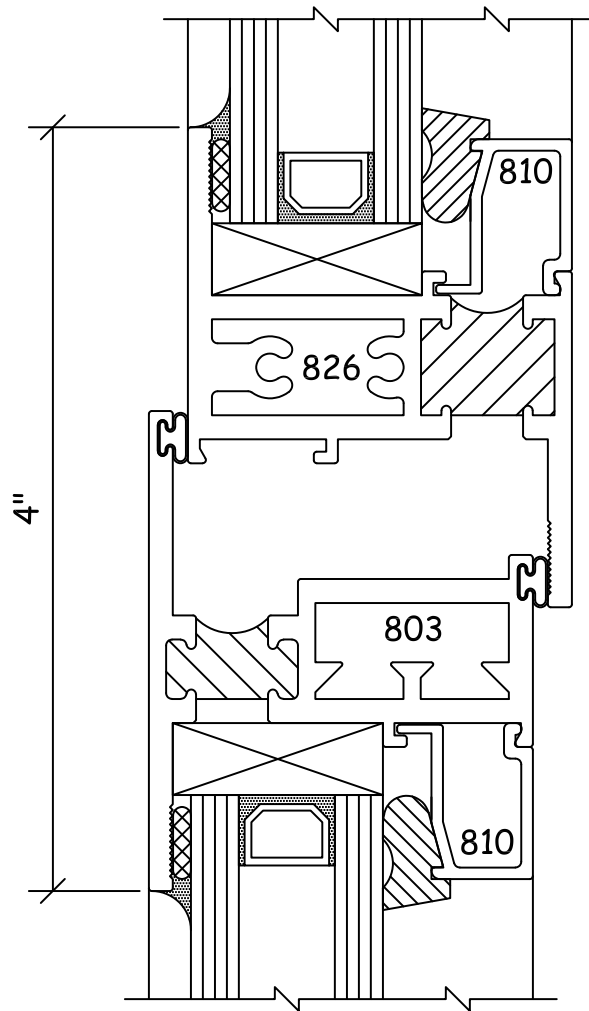
9 HORIZONTAL MUNTIN 8D5
